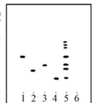
图 1 血栓通注射液 TLC 图
